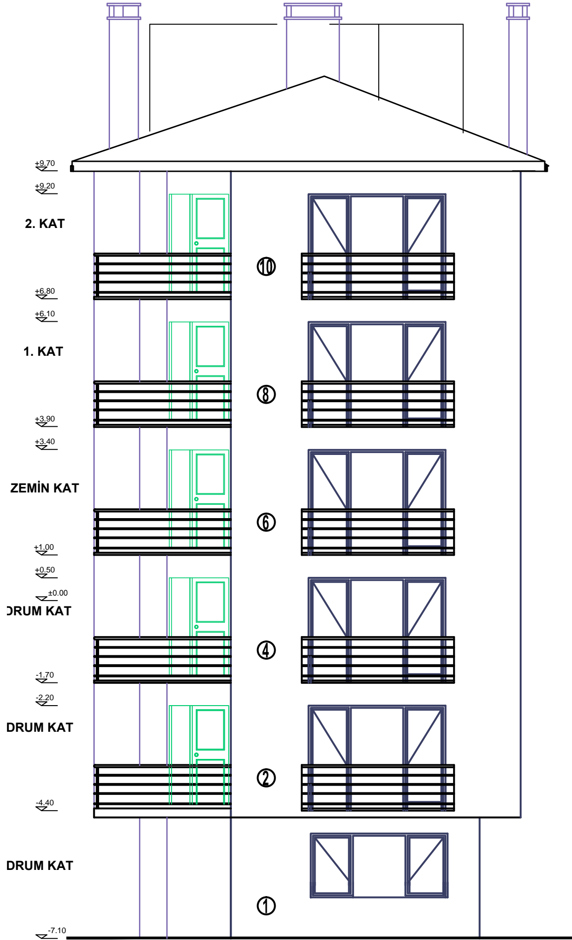
ÖN CEPHE Ö:1/50
