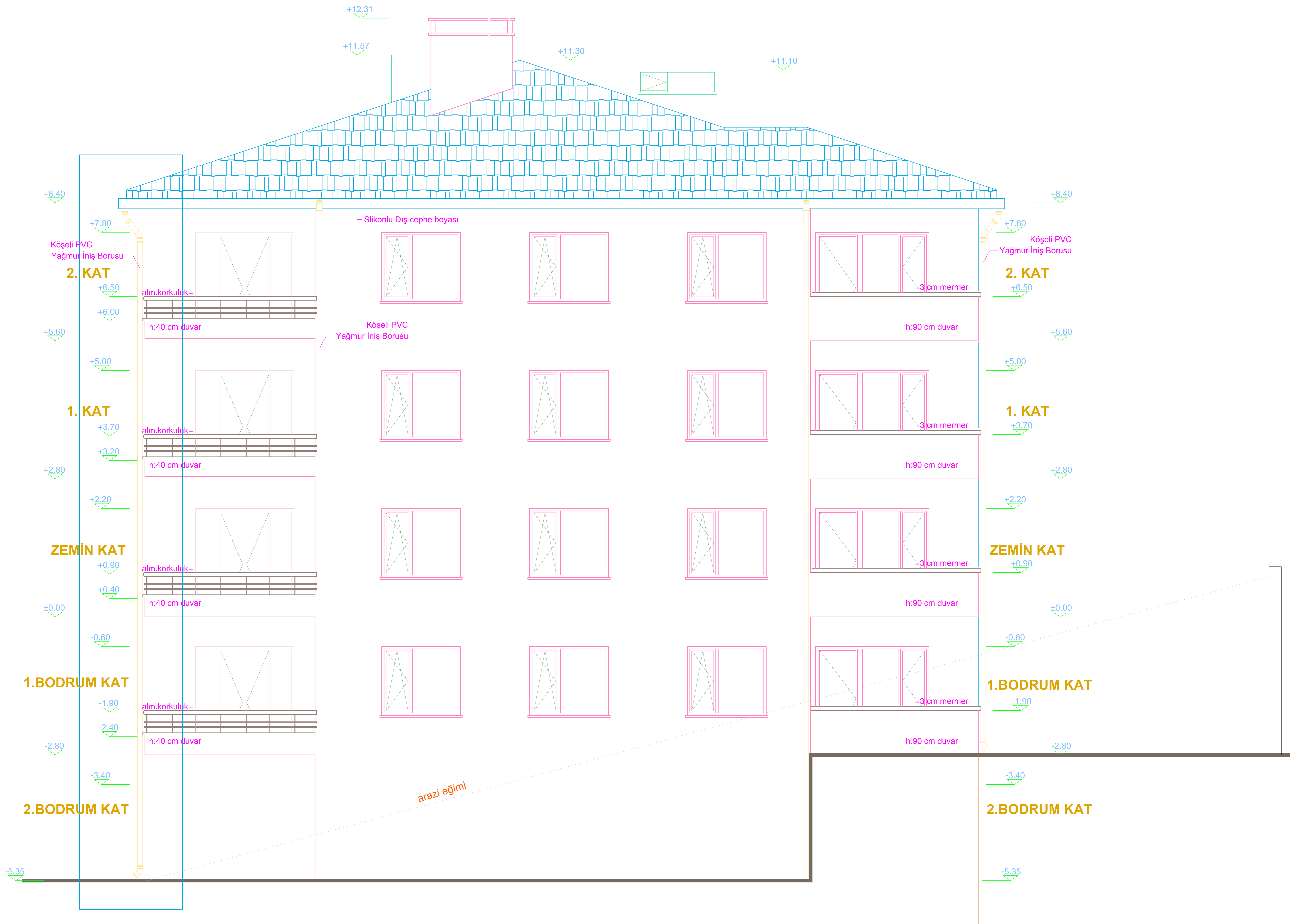
A1 BLOK SAĞ YAN CEPHE 1 / 50
