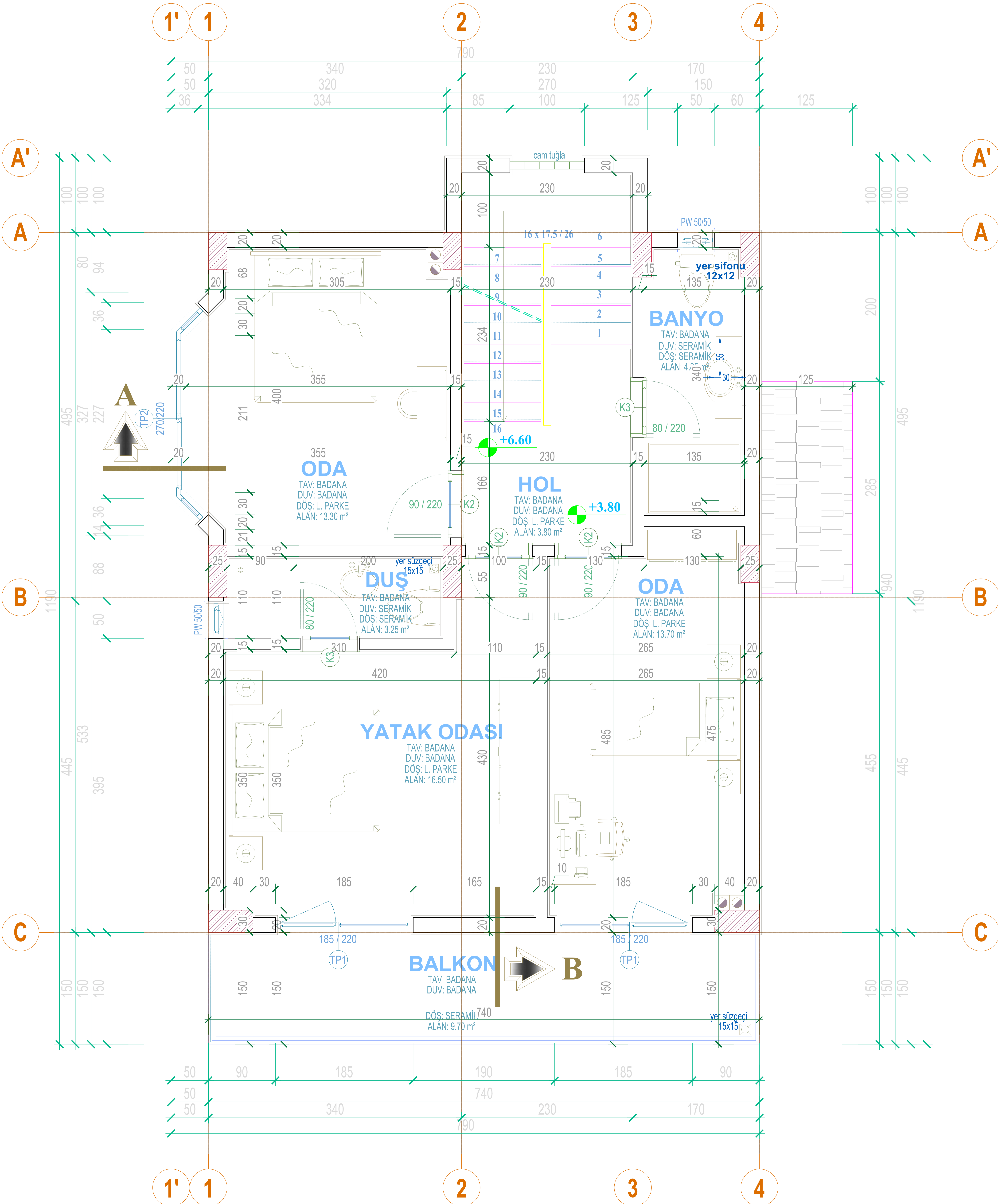
1. KAT PLANI 1 / 50
