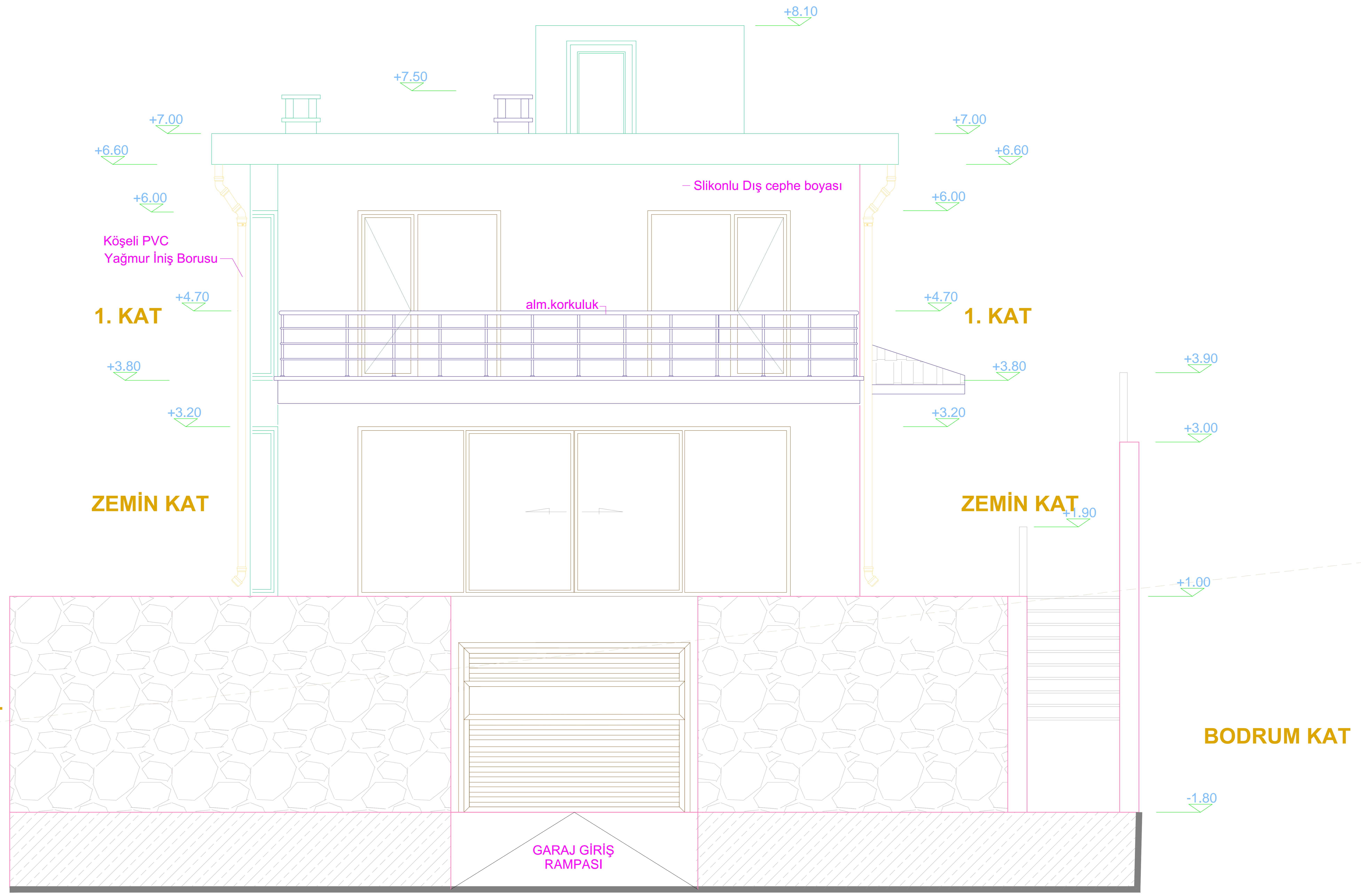
ÖN CEPHE 1 / 50
